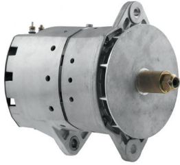
812-36111 12V 170A hinge MOUNT
